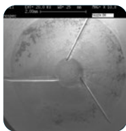
Tangentialschlitze der Düse in Makroaufnahme mit Clean up
